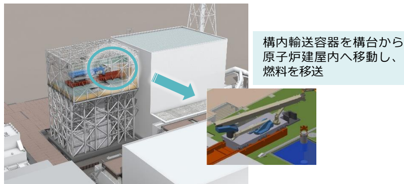
燃料取り出し用構台イメージ
