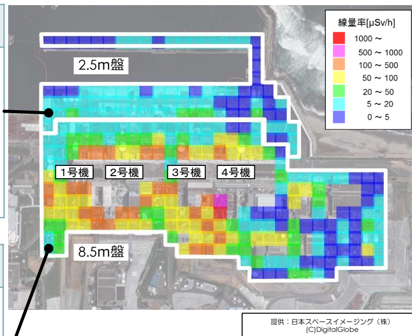
線量分布 (30mメッシュ：胸元高さ)
