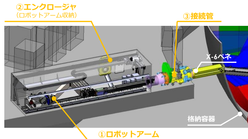
試験的取り出し装置の概要
