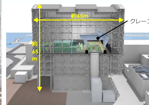
燃料取り出し時のイメージ
