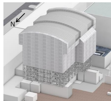
大型カバー設置時イメージ
